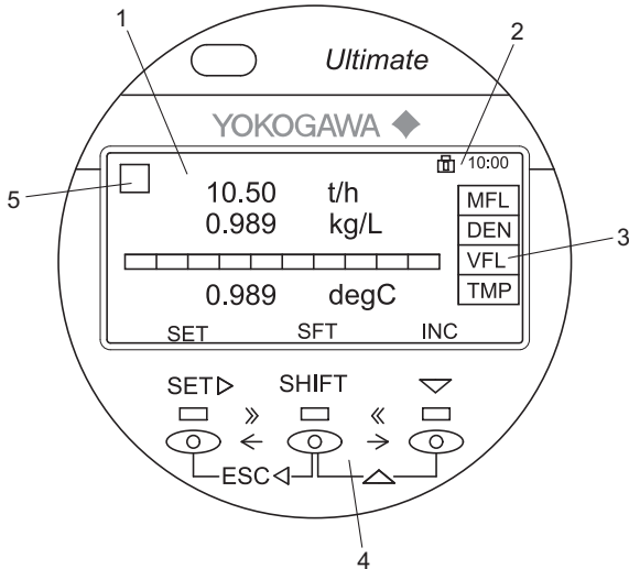
Fig. 37: Display layout
